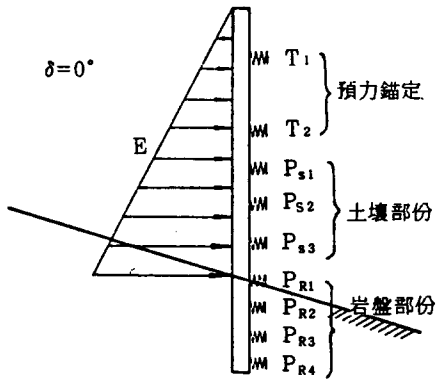
圖十二 彈性法
