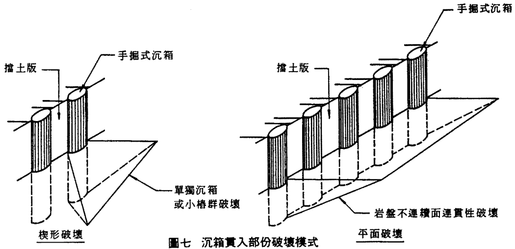
圖七 沉箱貫入部份破壞模式
