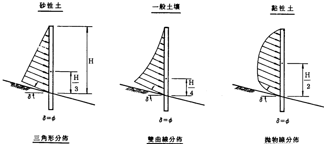
圖六 土壓力分佈形狀
