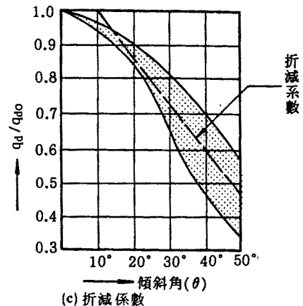
圖九 沉箱基底承載力 (摘自前田、良刀1986)
