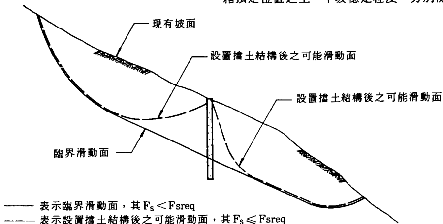
圖四 沉箱擋土牆位置示意圖
