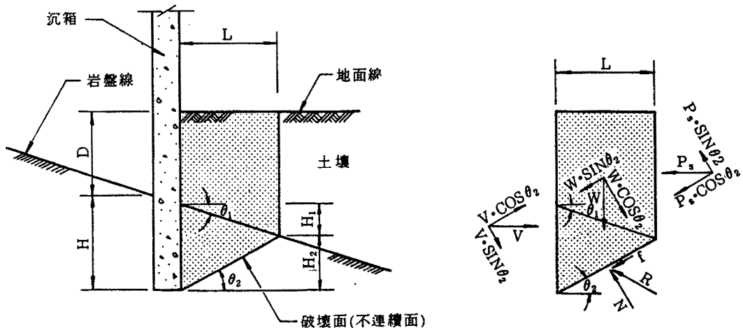
圖八 沉箱極限側向抵抗力解析圖
