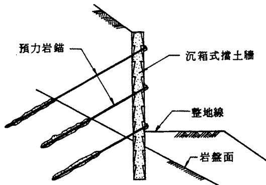
圖二 配置預力岩錨之沉箱式擋土牆
