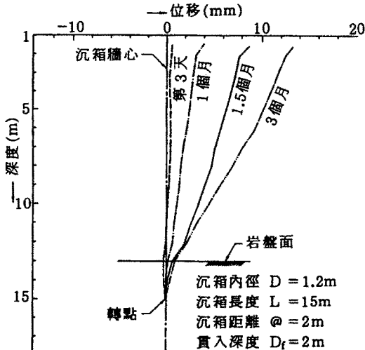
圖十 沉箱內傾斜儀觀測結果
