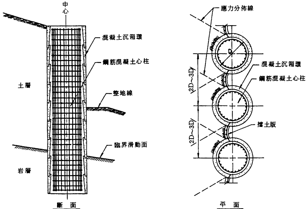
圖一 沉箱擋土牆詳圖
